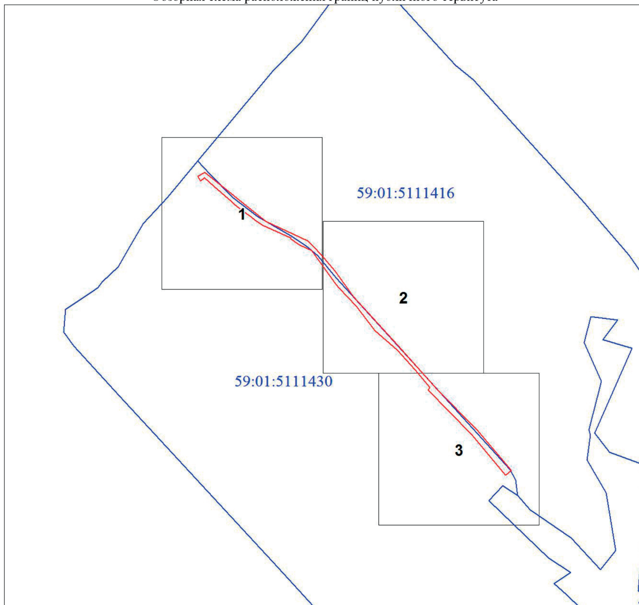
Обзорная схема расположения границ публичного сервитута
